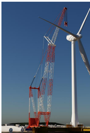
リングリフトクレーン
